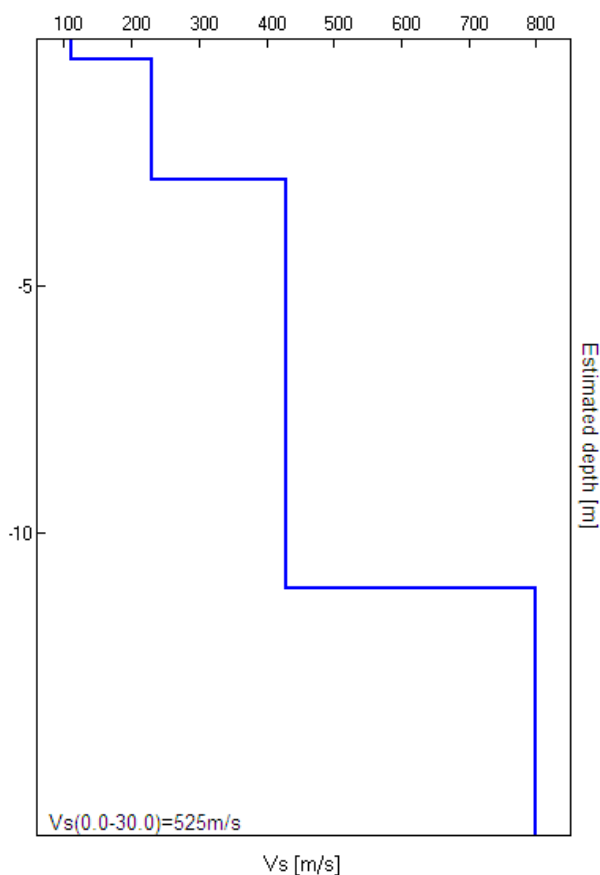
figura n. 9: sismostratigrafia
