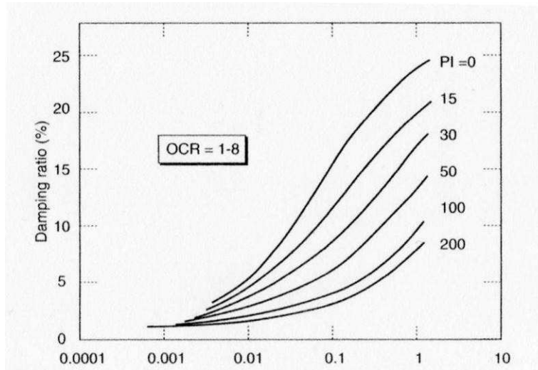
figura n. 17: influenza della plasticità sul coefficiente di smorzamento viscoso
